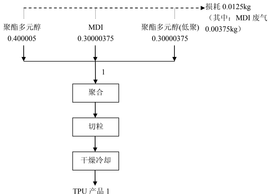
图 3.2-2 莘塍厂区 3.0 万吨/年 TPU 项目生产物料平衡 (单位: t/t 产品)
