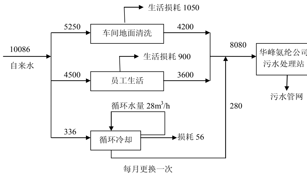
图 4.5-5 本次新增 2.8 万吨/年 TPU 项目水平衡简图 (单位: t/a)
