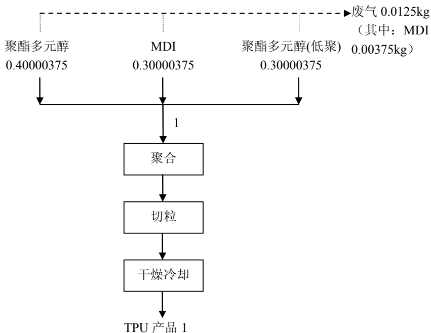
图 4.5-4 技改后 2.8 万吨/年 TPU 项目生产物料平衡（单位：t/t 产品）
