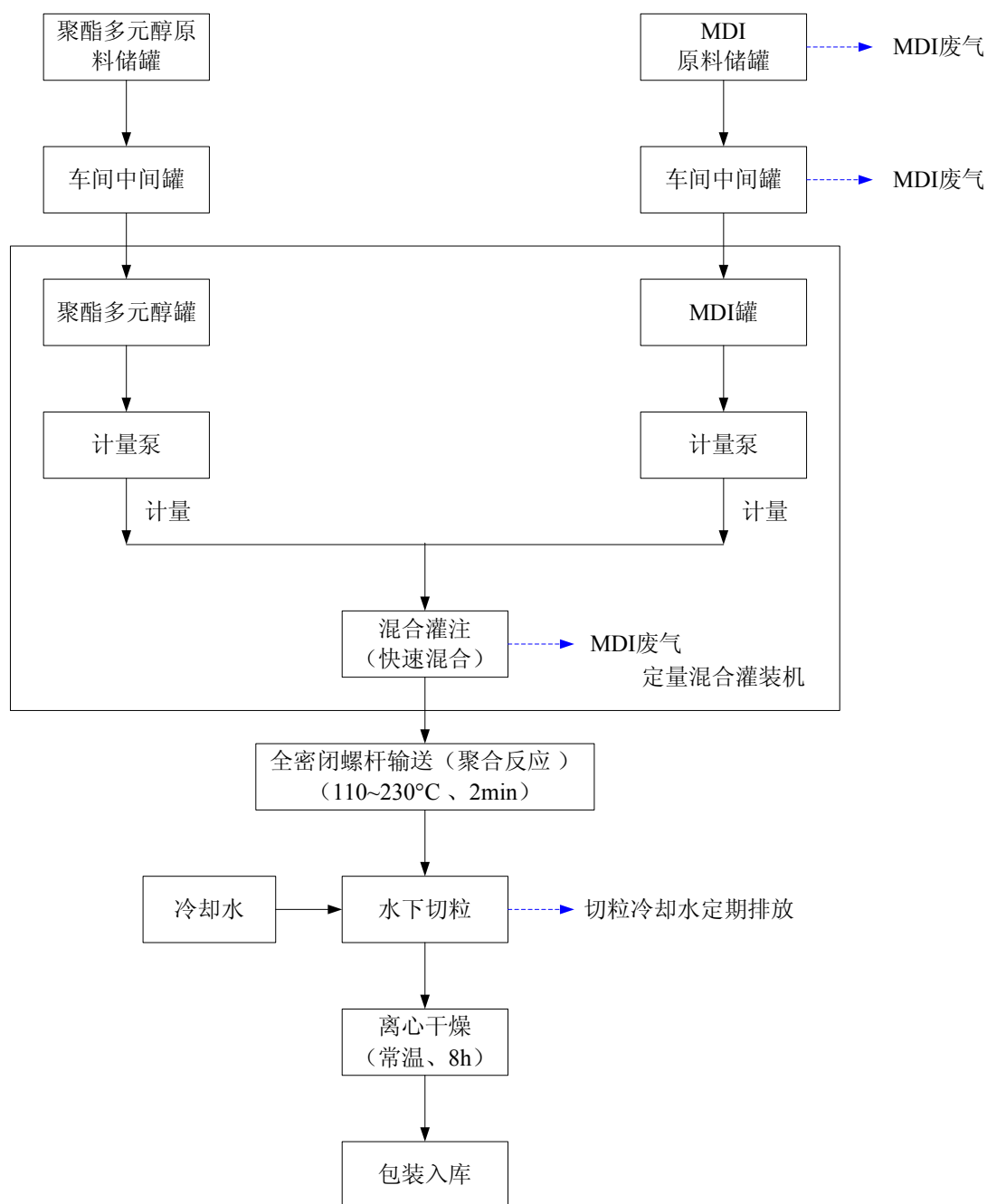
图 4.5-1 技改后热熔胶生产工艺流程图
