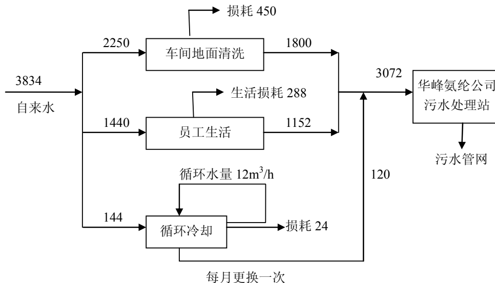
图 3.3-1 东山厂区 1.2 万吨/年 TPU 项目水平衡简图（单位：t/a）
