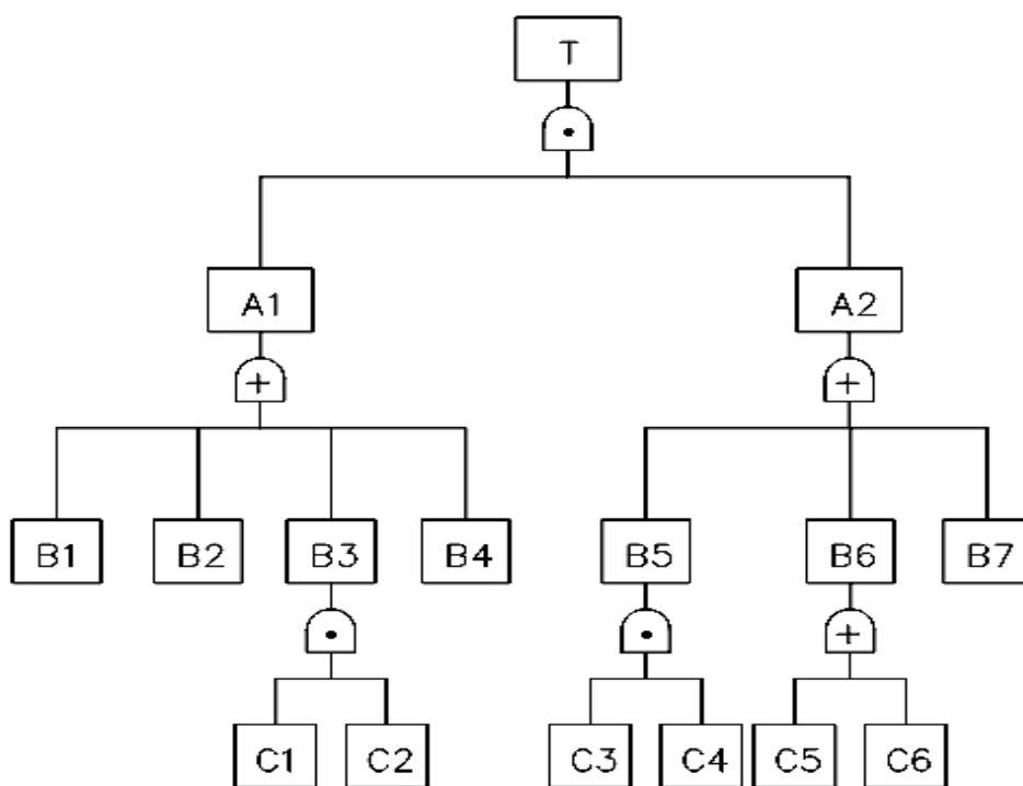
图 7.3-1 事故树
