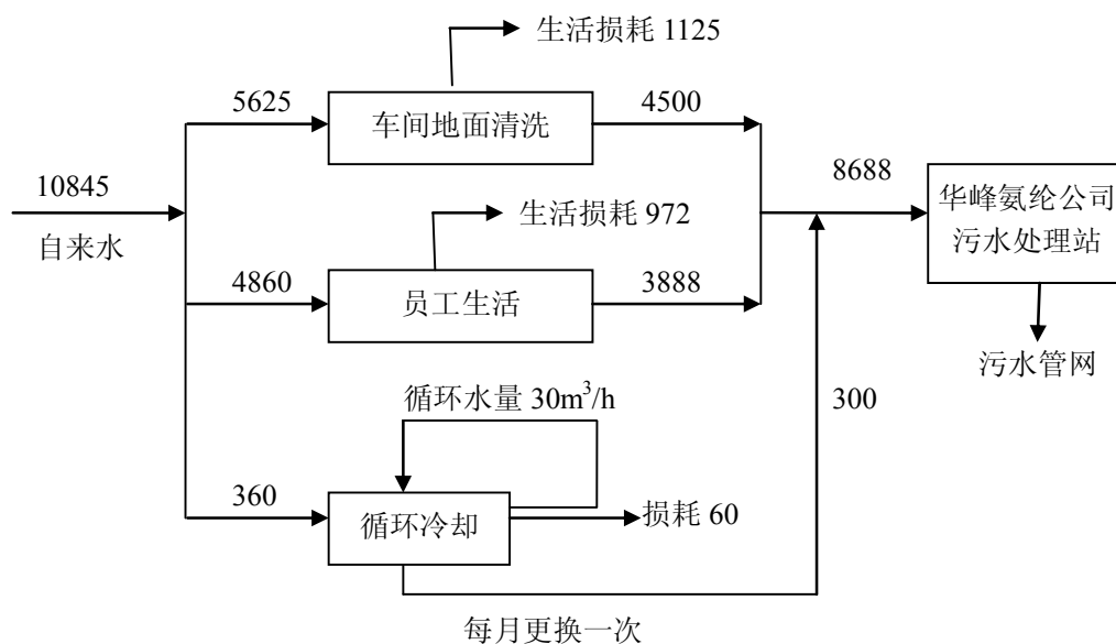
图 4.5-6 技改后莘滕厂区项目水平衡简图 (单位: t/a)
