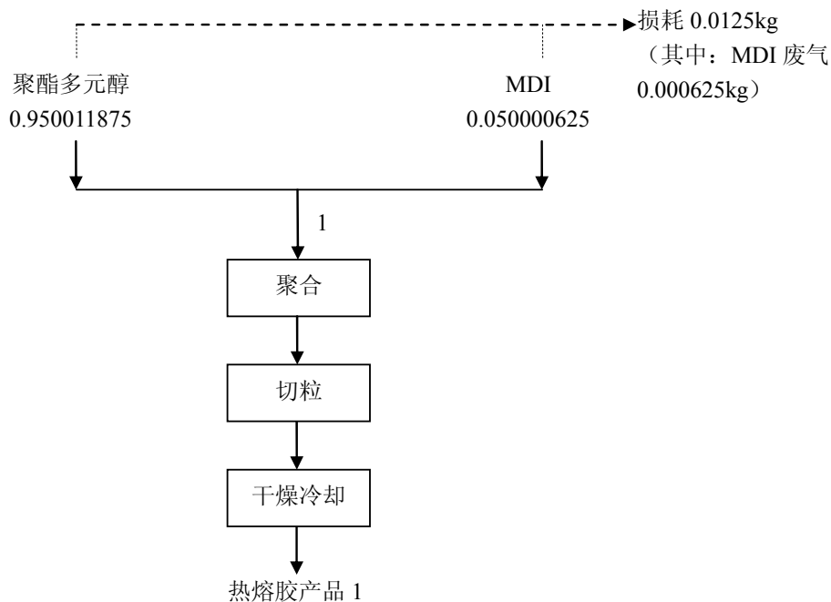
图 4.5-2 本次新增 2000 吨/年热熔胶项目生产物料平衡（单位：t/t 产品）
