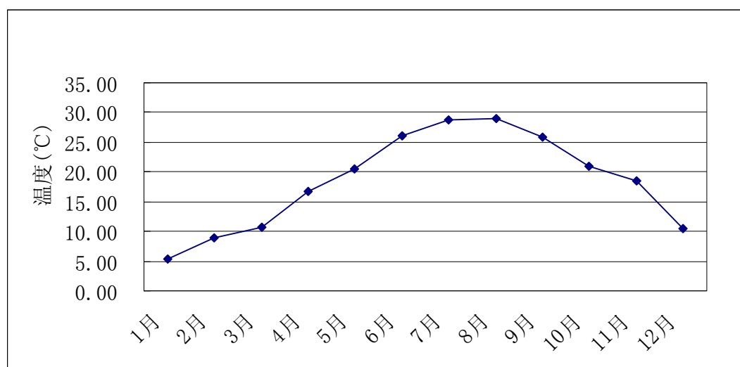
图 6.2-1 年平均温度月变化曲线图
