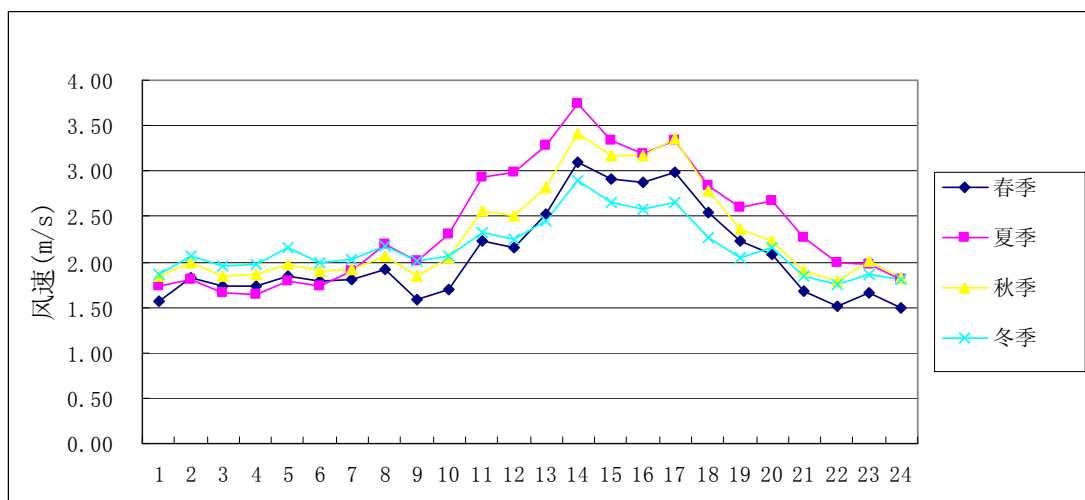
图 6.2-3 季小时平均风速日变化曲线
