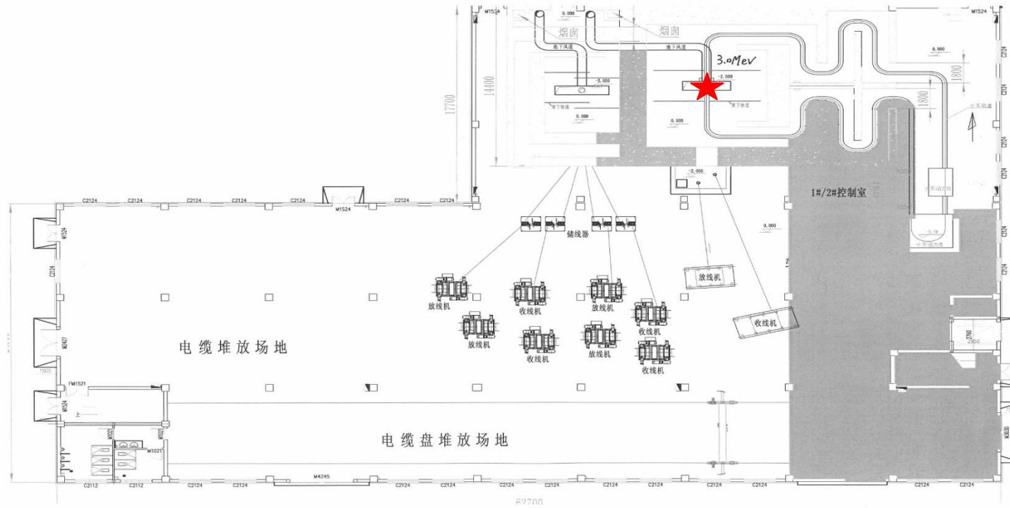
图 2-3 乐清市华仪电缆附件有限公司辐照加工车间平面布置示意图
