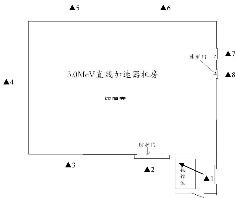
3.0MeV 直线加速器机房一楼平面图
