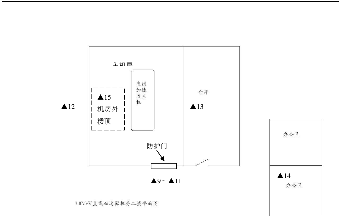
图 5-1 加速器机房周围监测点位示意图
